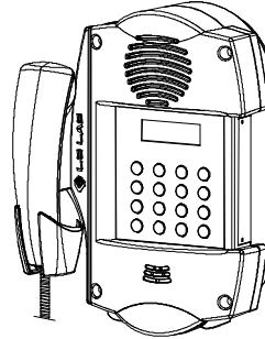
TLS 229 A1C9FGL телефон "свободные руки", с клавиатурой 14 кнопок, с трубкой, с дисплеем и лампой вспышкой
