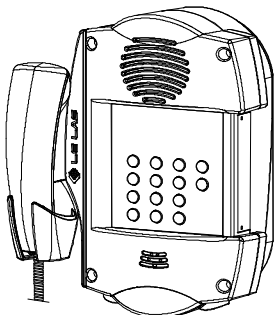
TLA 229 A1C9FG телефон с трубкой со звонком "пьезо", клавиатурой 14 кнопок, лампа- вспышка при вызове
