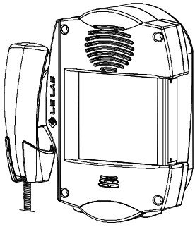
TLC 229 A1 телефон с трубкой со звонком "пьезо"
